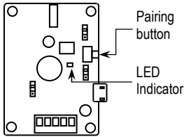
Sensor (RM-R100-TLQ)
